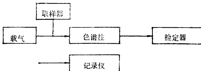
图1 电子级氢中痕量氧+氩、氮测定流程图
